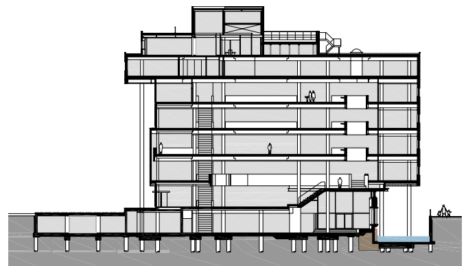
dwarsdoorsnede
