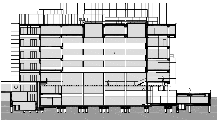
langsdoorsnede
